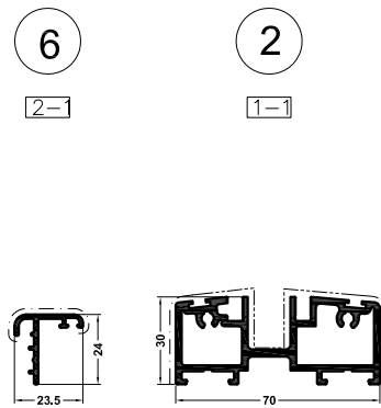
DV56 omtrek: 131mm DV70 omtrek: 347mm
