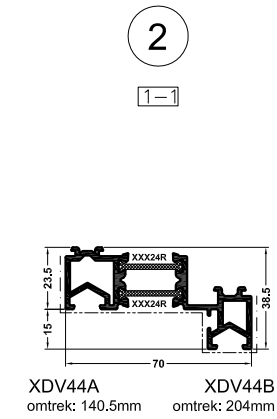
DV44 omtrek: 320.9mm
