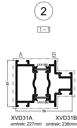
DV31 omtrek: 323mm
