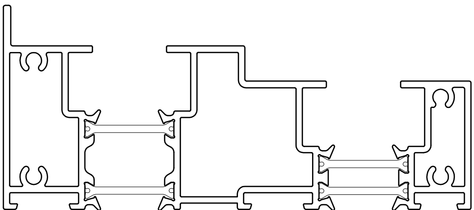
VS112 Slim Jamb Section
