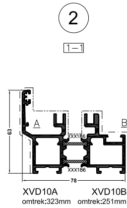
DV10 omtrek: 488mm
