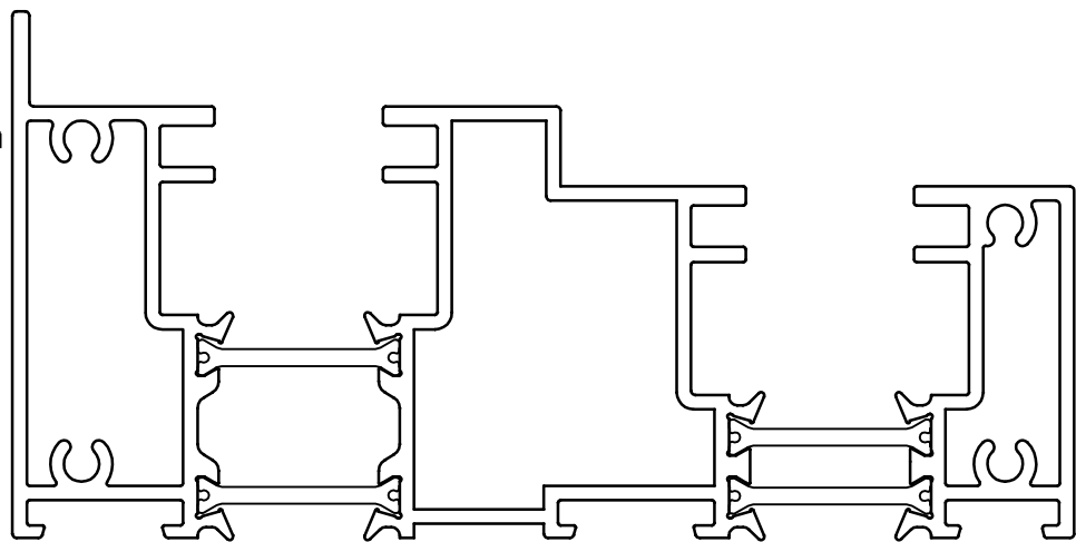
VS012 Jamb Section
