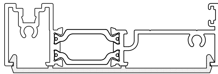
GSL1145 External Jamb PVC Clip Plate
