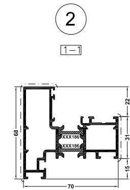
DV121 omtrek: 437.7mm
