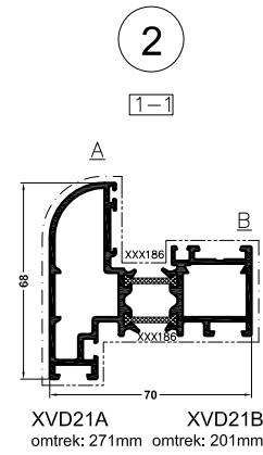
DV21 omtrek: 389mm
