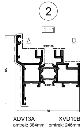
DV13 omtrek: 586.12mm
